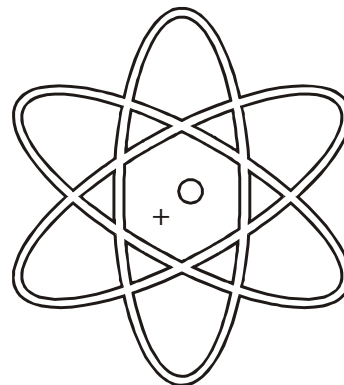
Modelo de Sommerfeld ( )
